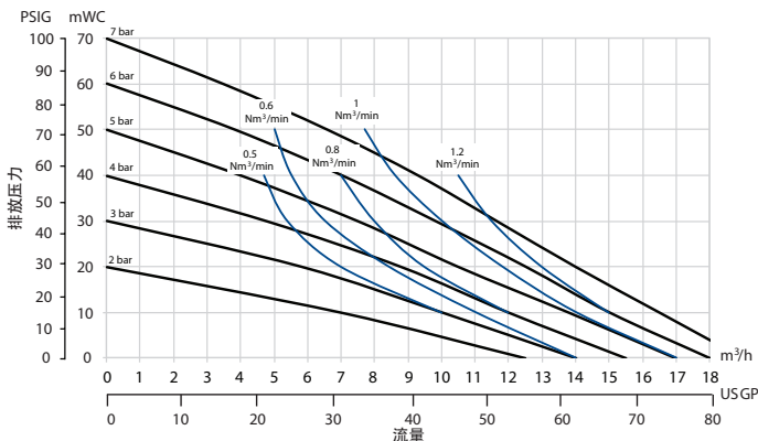
D150性能曲线
