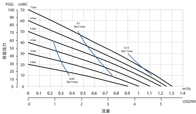
D038性能曲线
