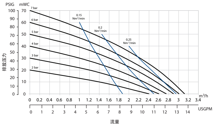
D050性能曲线
